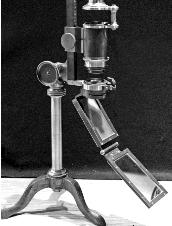
Fig. 5a : Dispositif imaginé par Émile Bertrand pour les études en lumière convergente (Musée ENSMP). Photo José-Marcio Martins da Cruz, École des mines, Paris.
