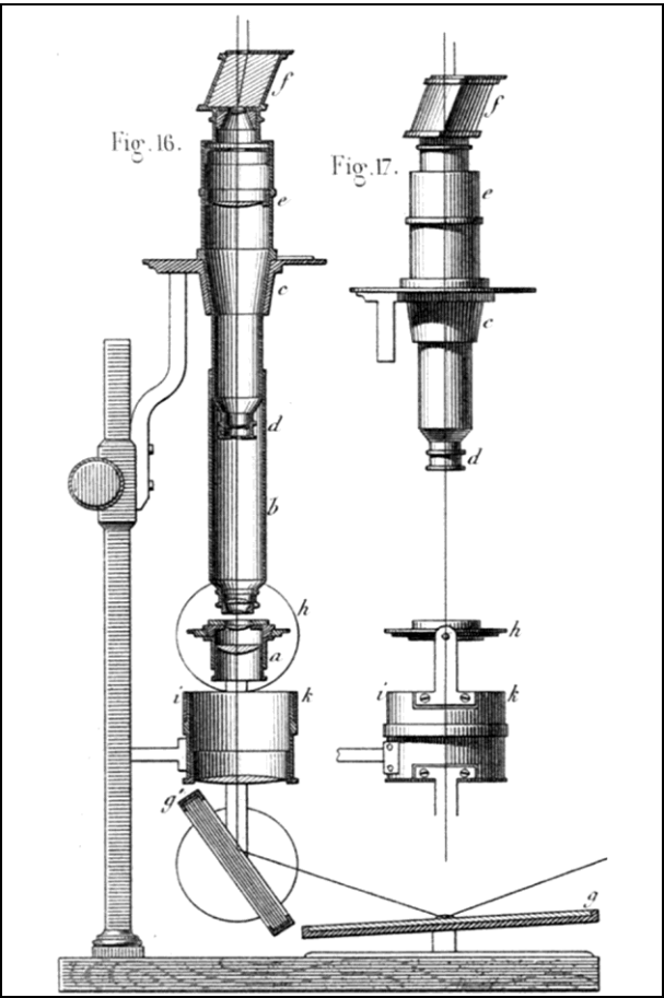
Fig. 1b : Schéma de principe du dispositif optique, in Claude Pouillet, Éléments de Physique expérimentale et de Météorologie , Atlas, Planche 45, L. Hachette et Cie, 1853.
